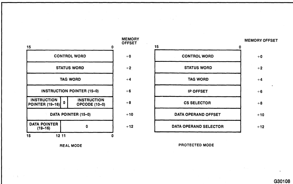
Figure 2-2. FSTENV/FLDENV Memory Layout
