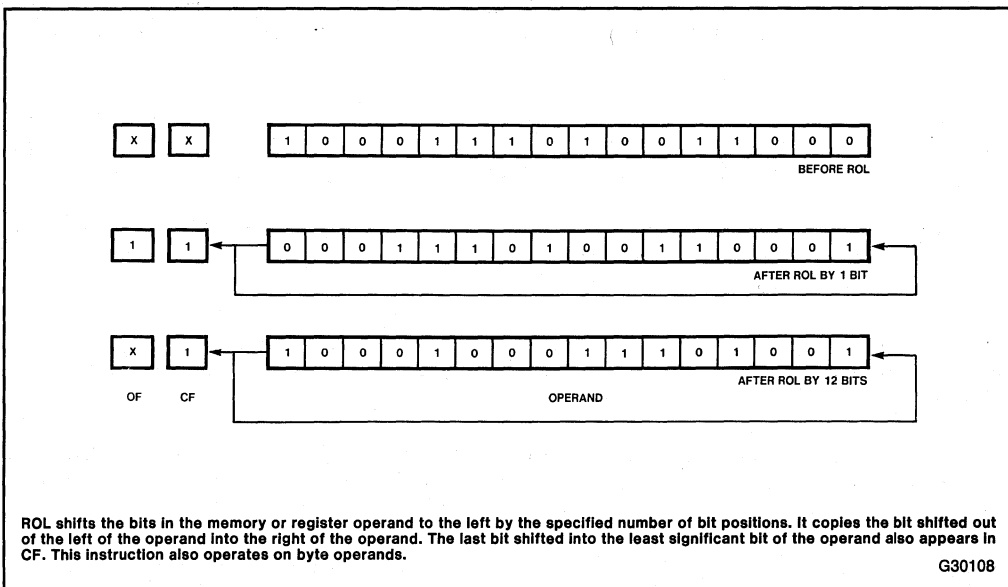
Figure 3-9. ROL
