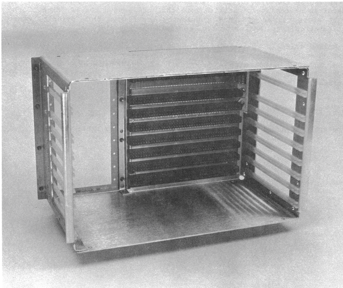
Figure 1-1. iSBC ® 608 Modular Cardcage/Backplane
